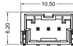
3pin
