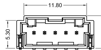
5pin
